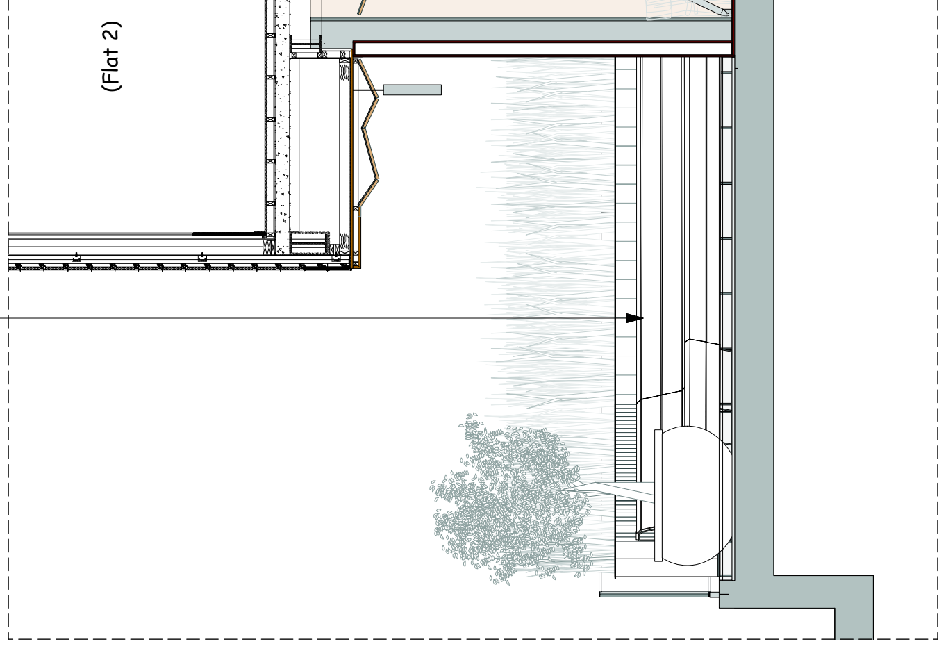
2 SECTION DD
