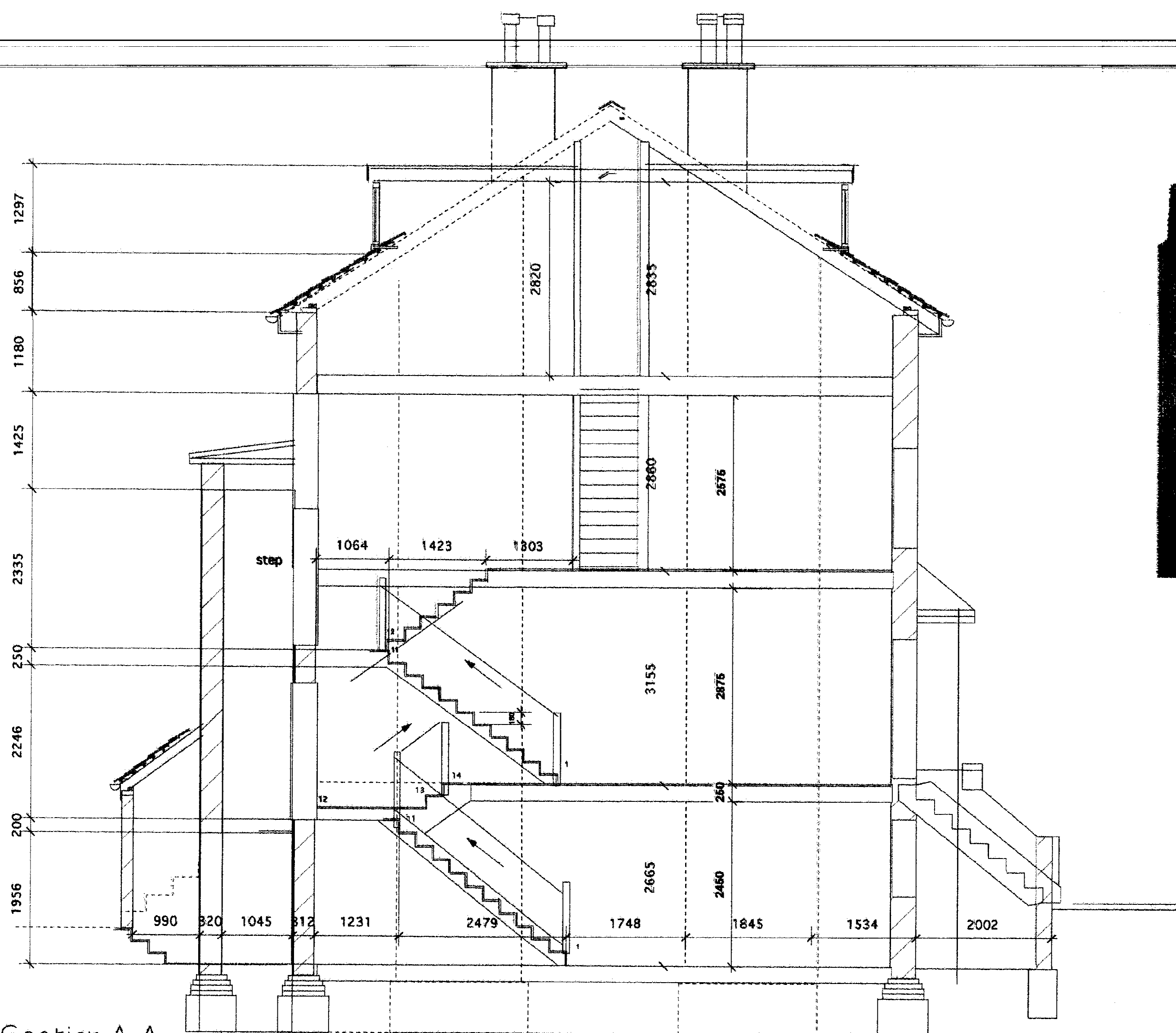
Section A-A
