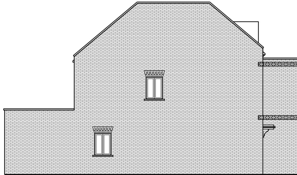
Side Elevation House Type F1
