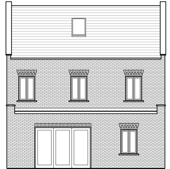
Rear Elevation House Type F1
