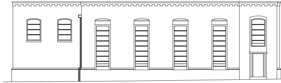
ELEVATION 8
