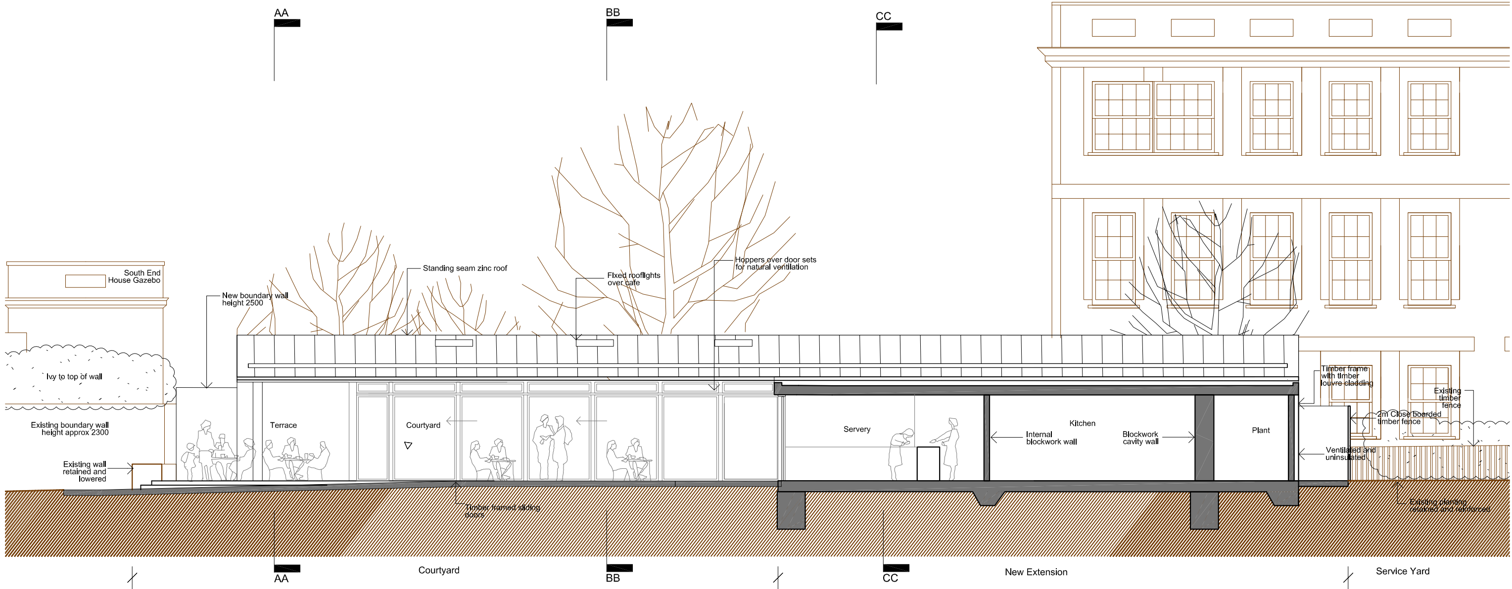
Section DD
