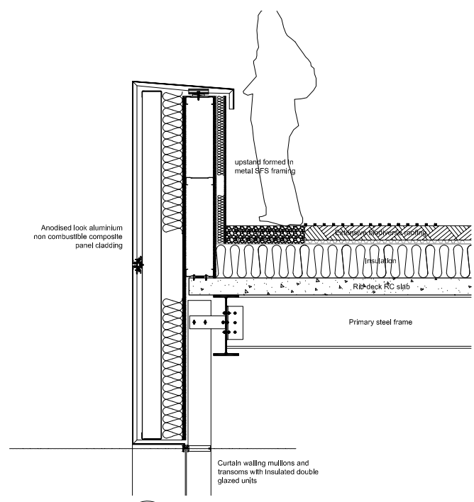
2 parapet 1:20
