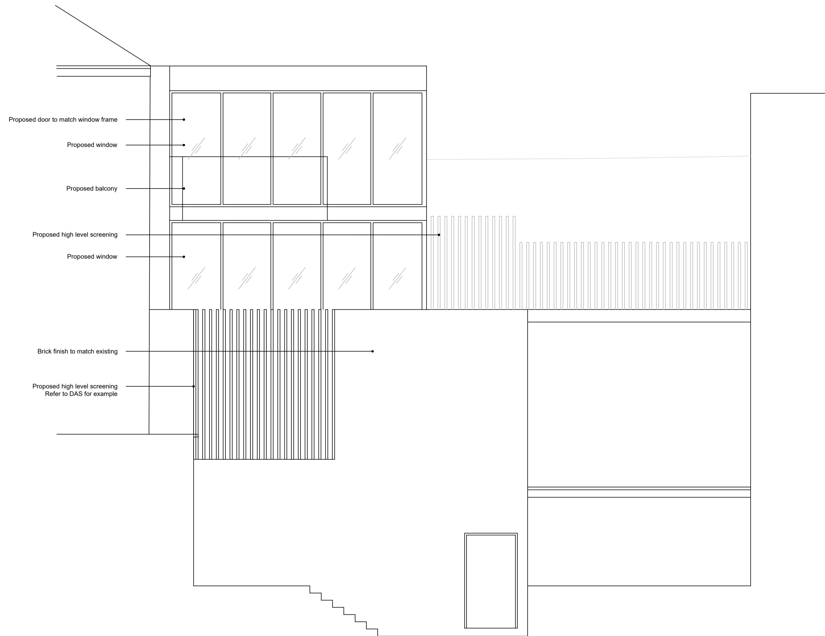
Rear Elevation Scale: 1/50
