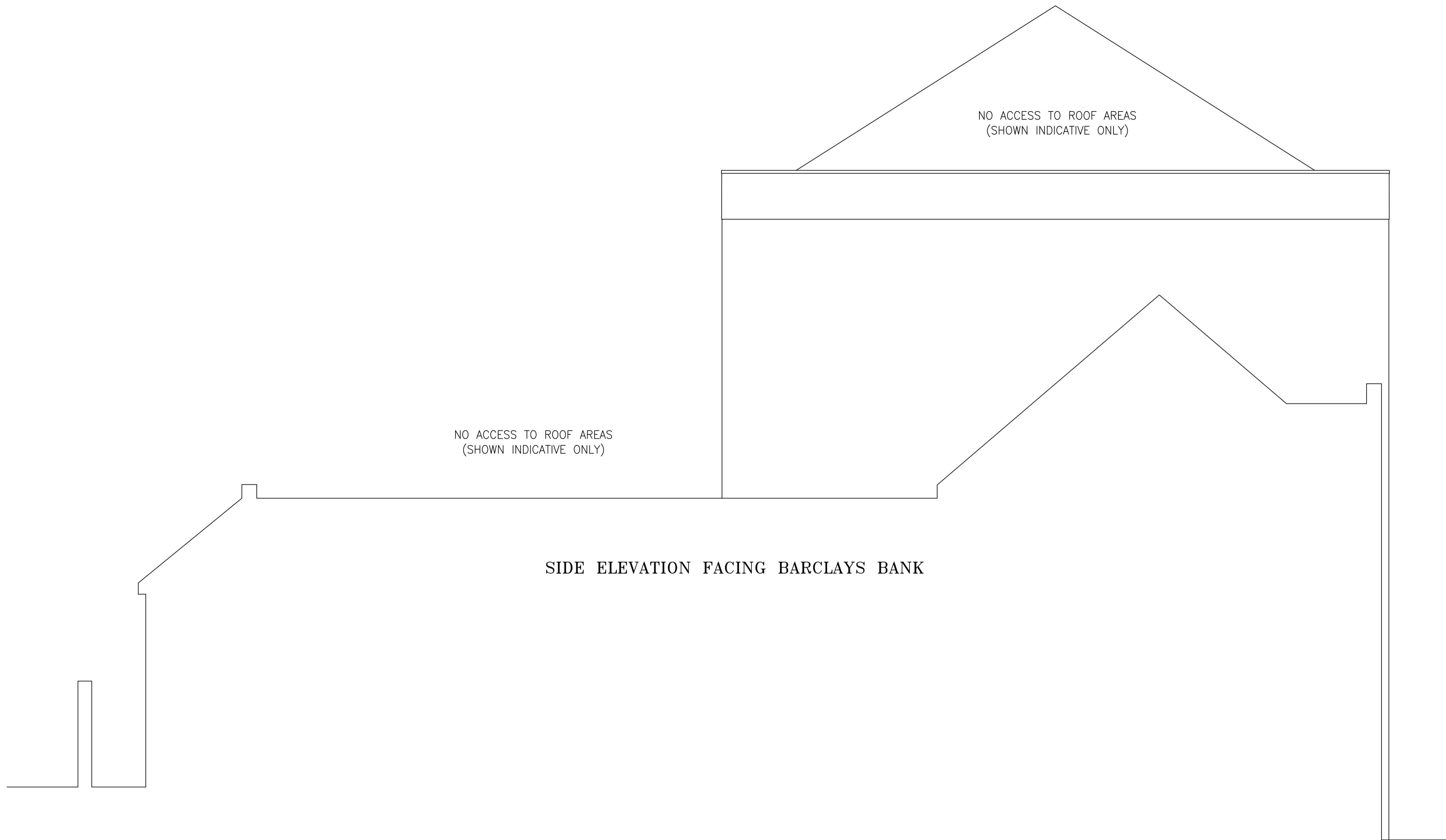
Side Elevation Scale: 1/50
