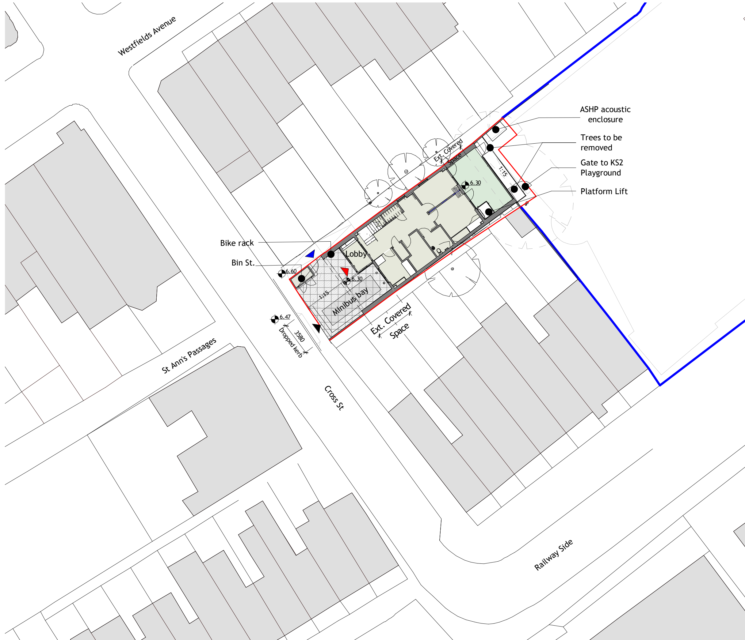
1 Site Layout 1 : 250
