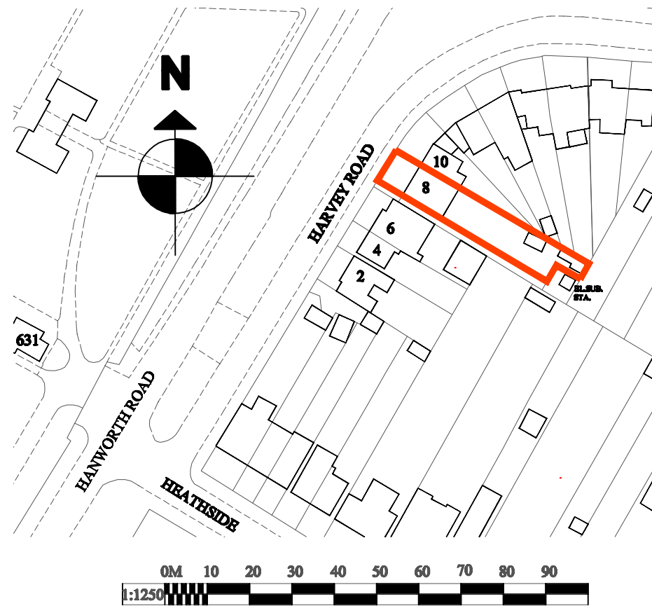
SITE PLAN 1:1250
