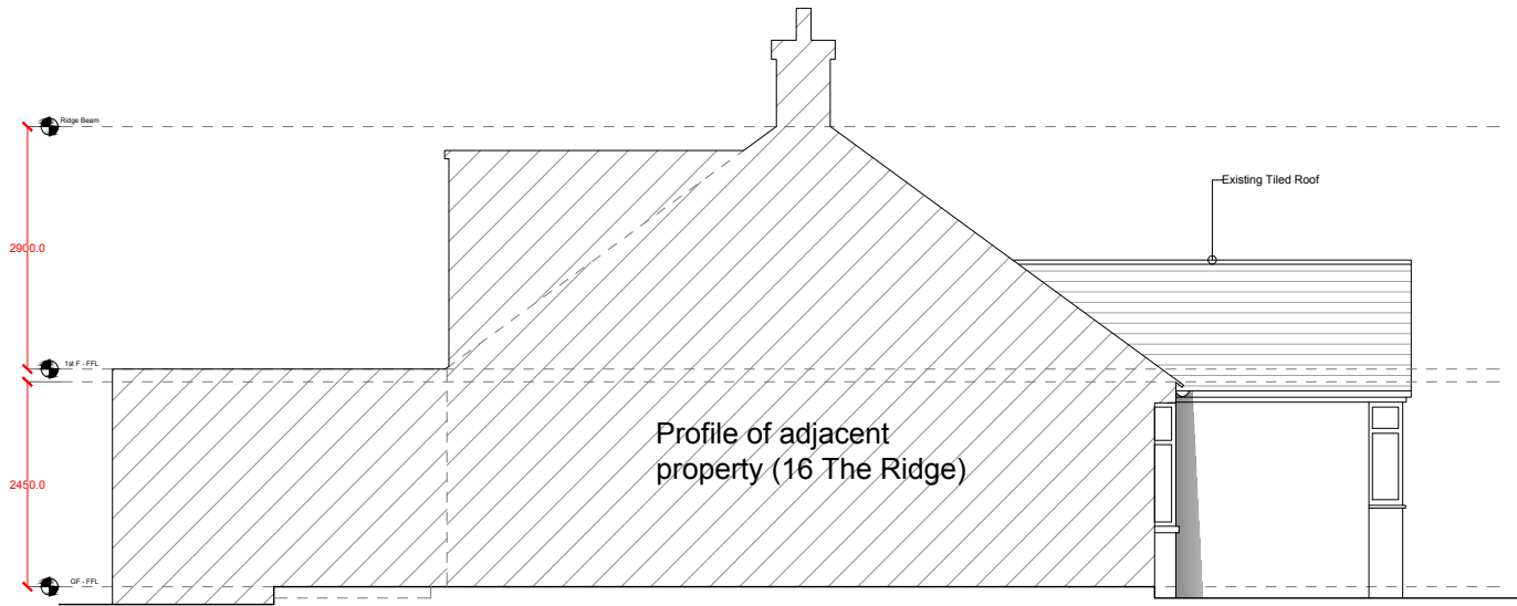
Existing Side Elevation (D)
