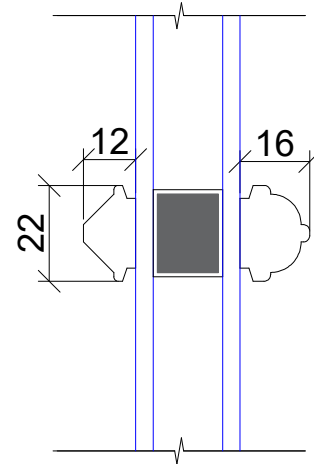
Glazing Bar
