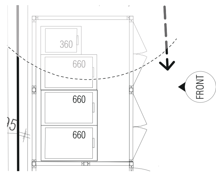
SITE A PLAN 1:50
