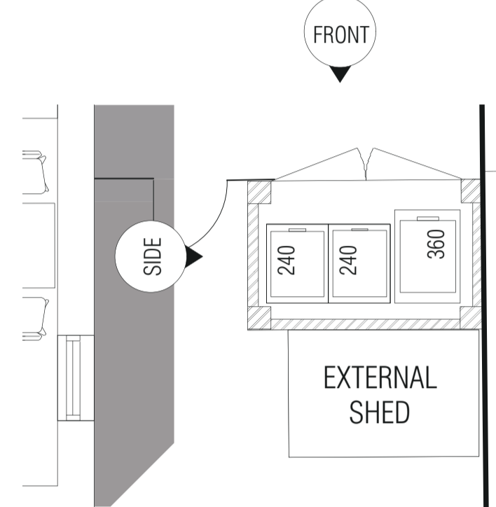
SITE B PLAN 1:50
