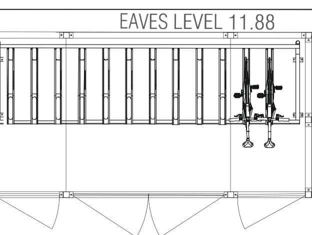
SITE B PLAN 1:50
