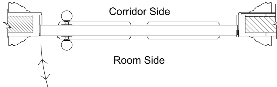
Section D-D
