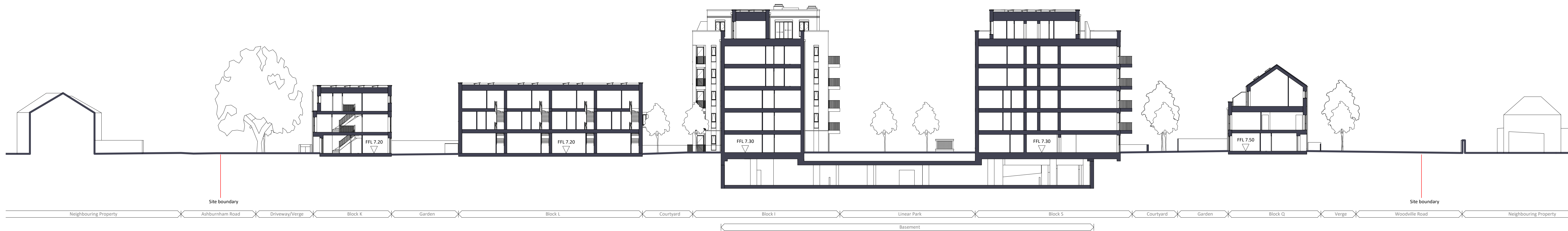
Site Section 4 1:250
