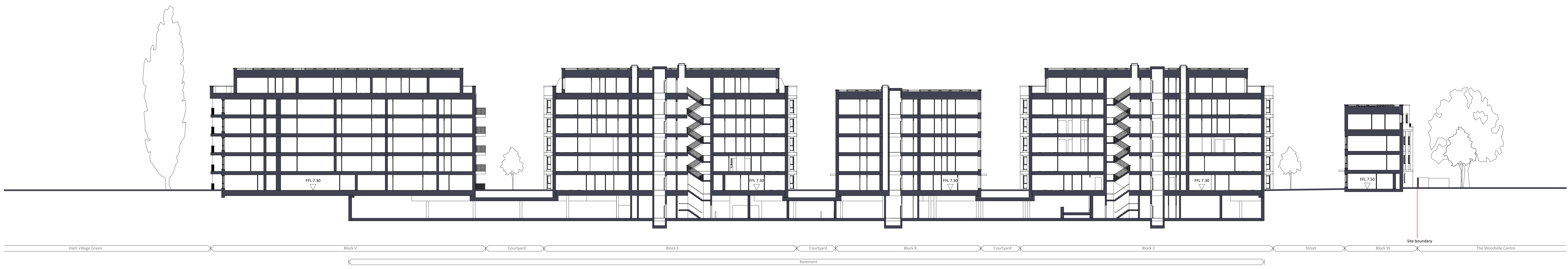
Site Section 1 1:250
