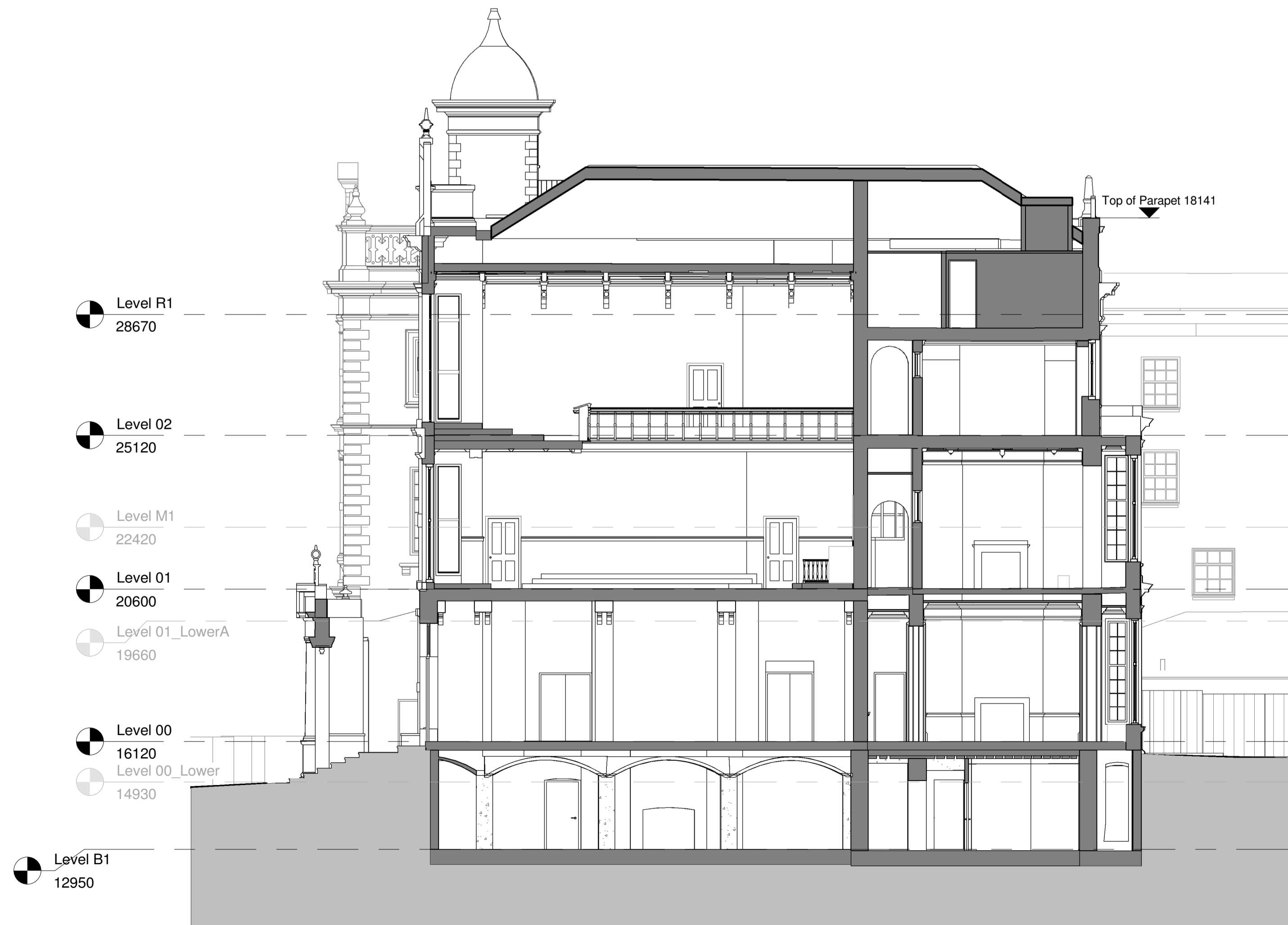
2 SECTION DD - EXISTING 1 : 100
