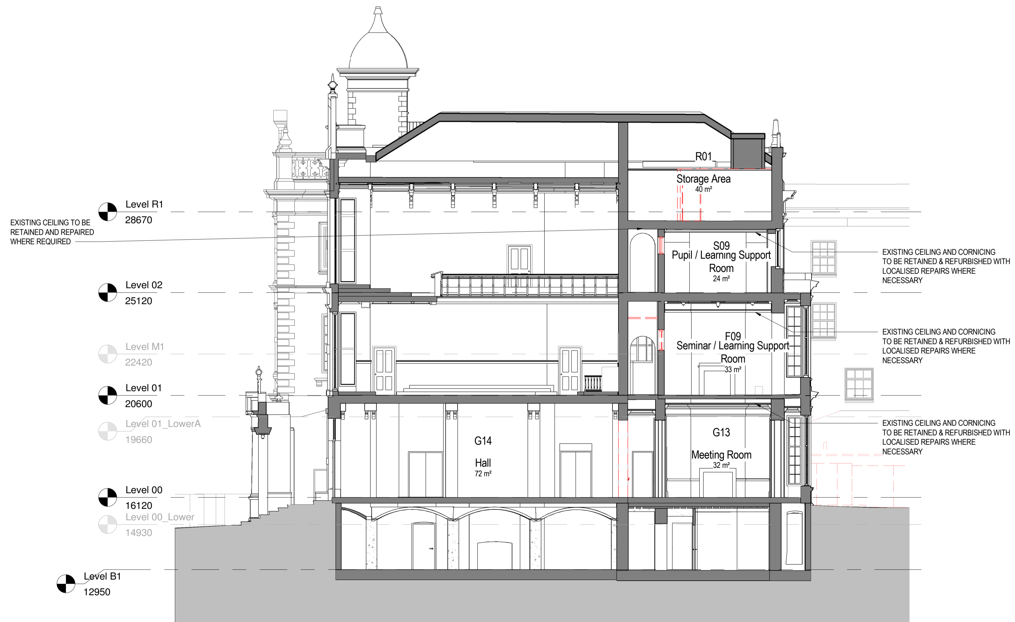
2 SECTION DD - DEMOLISHED 1 : 100
