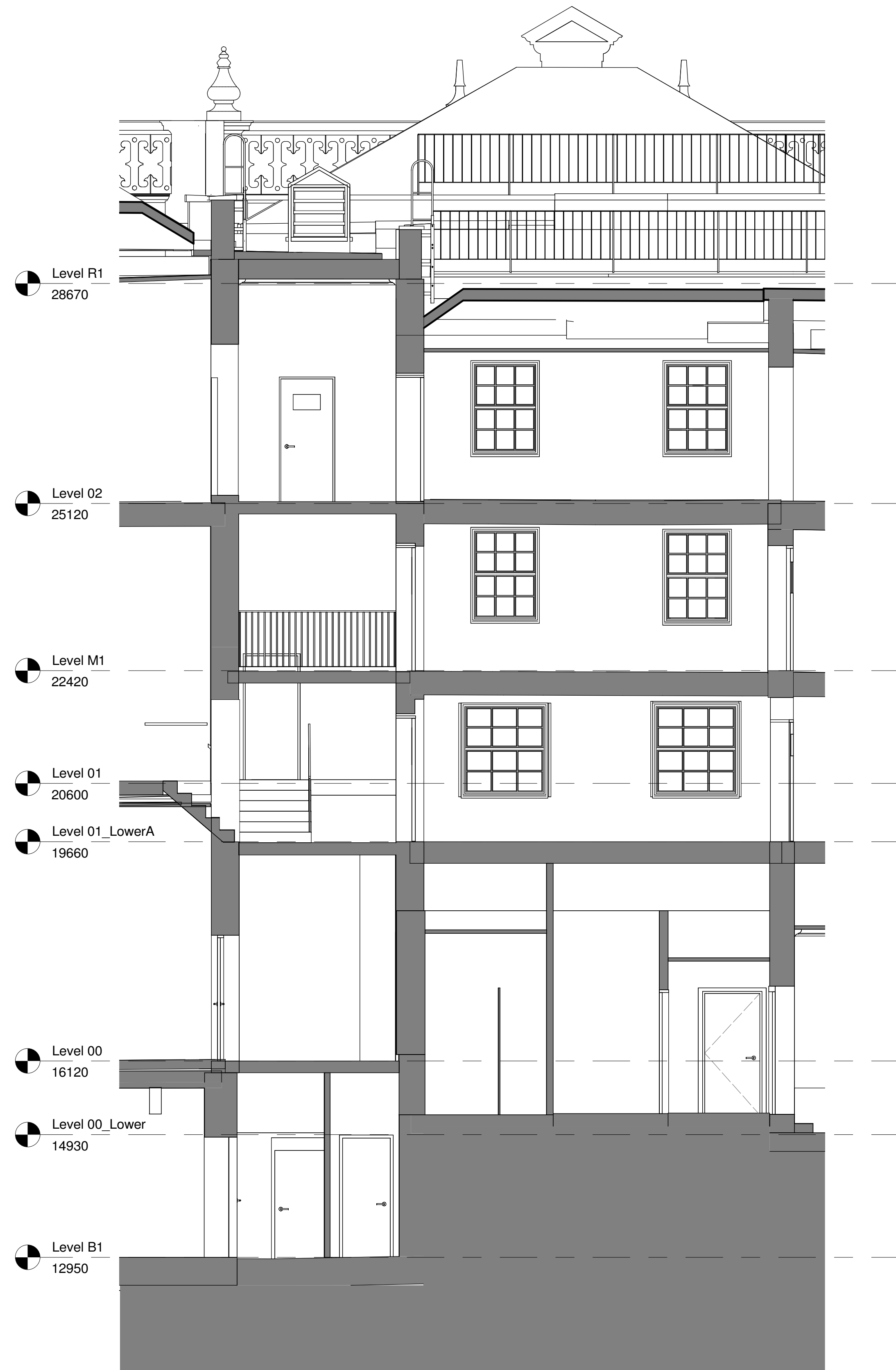
2 SECTION B STAIR - EXISTING 1 : 50
