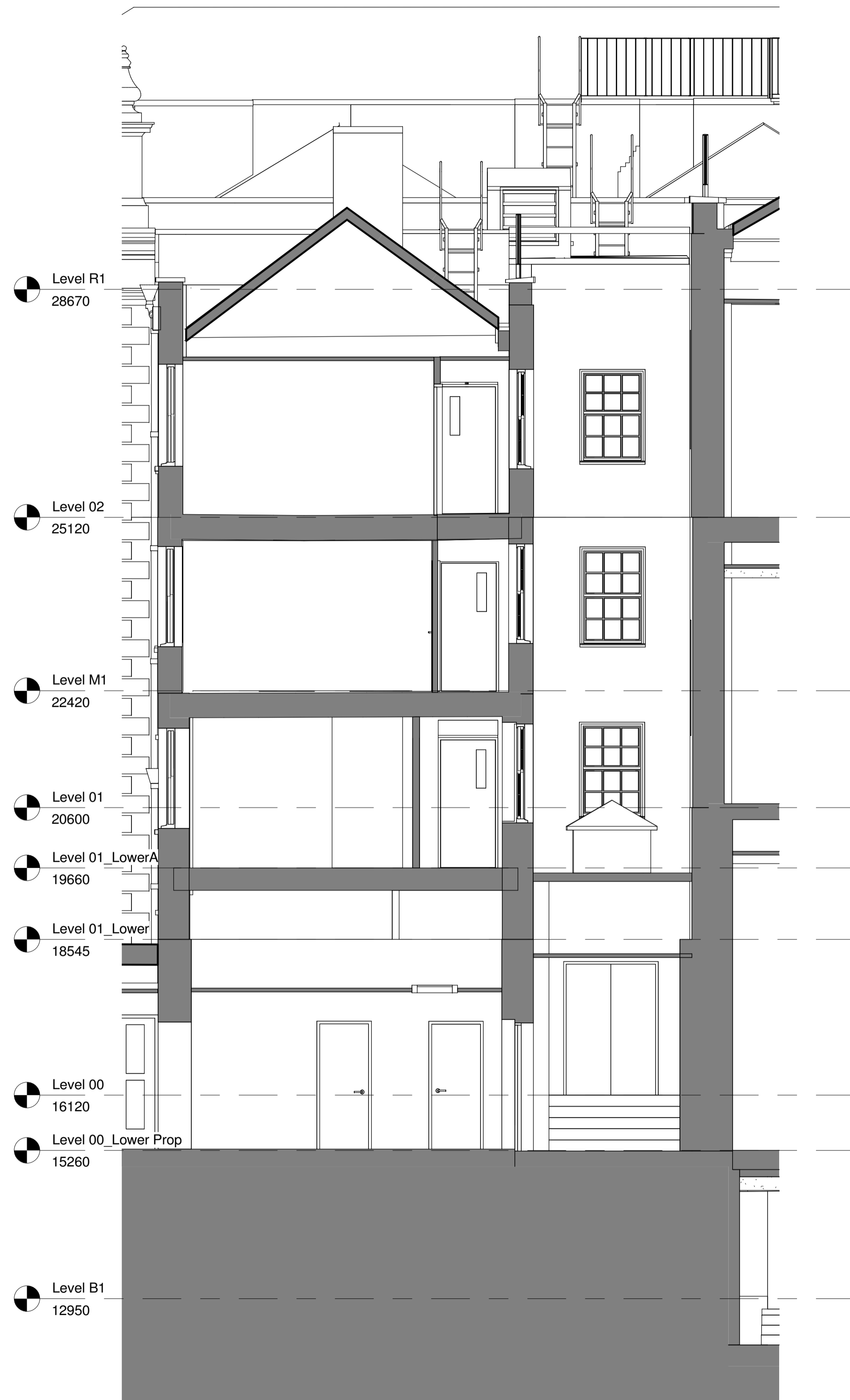
2 SECTION D STAIR - EXISTING 1 : 50
