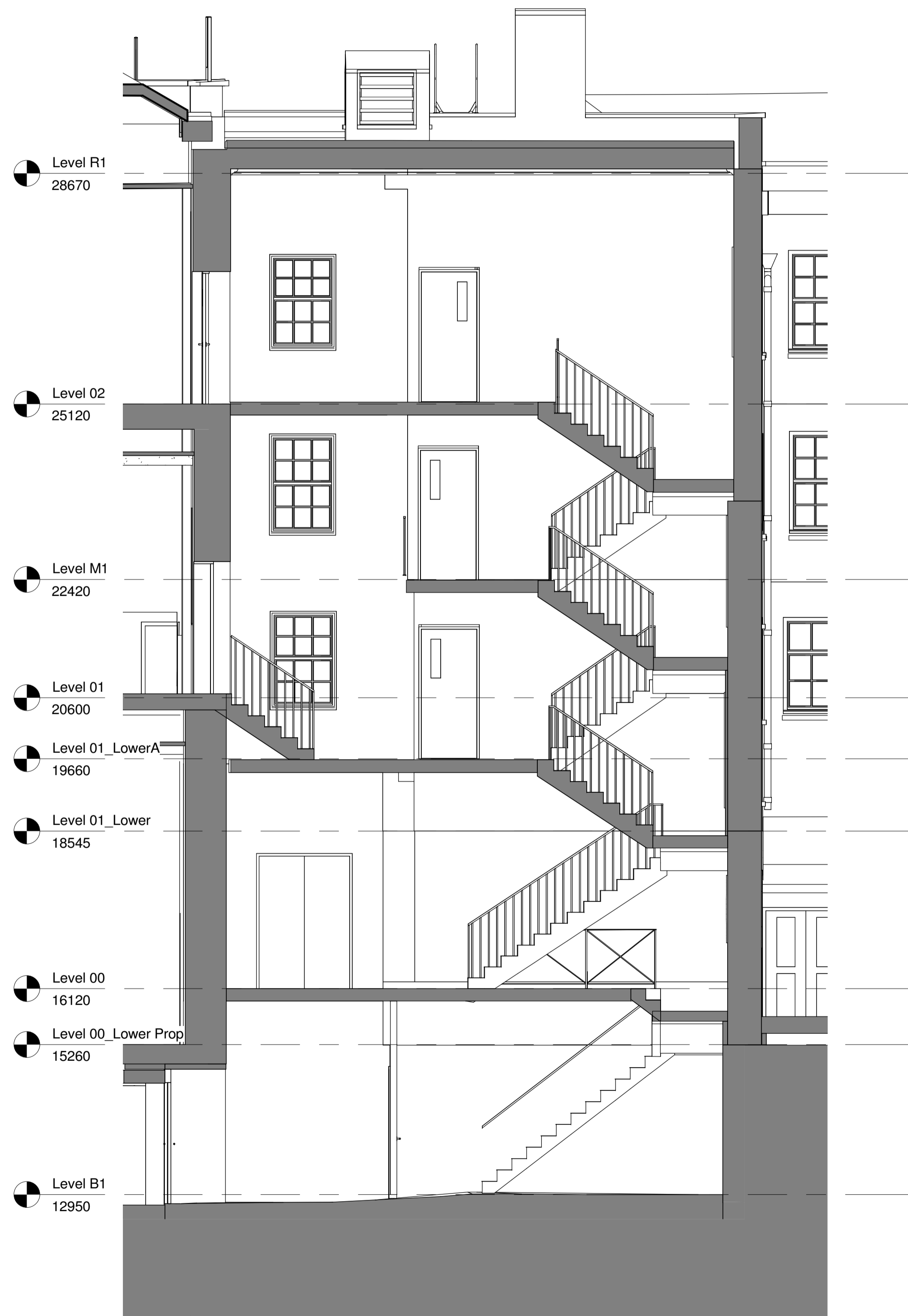
1 SECTION C STAIR - EXISTING 1 : 50
