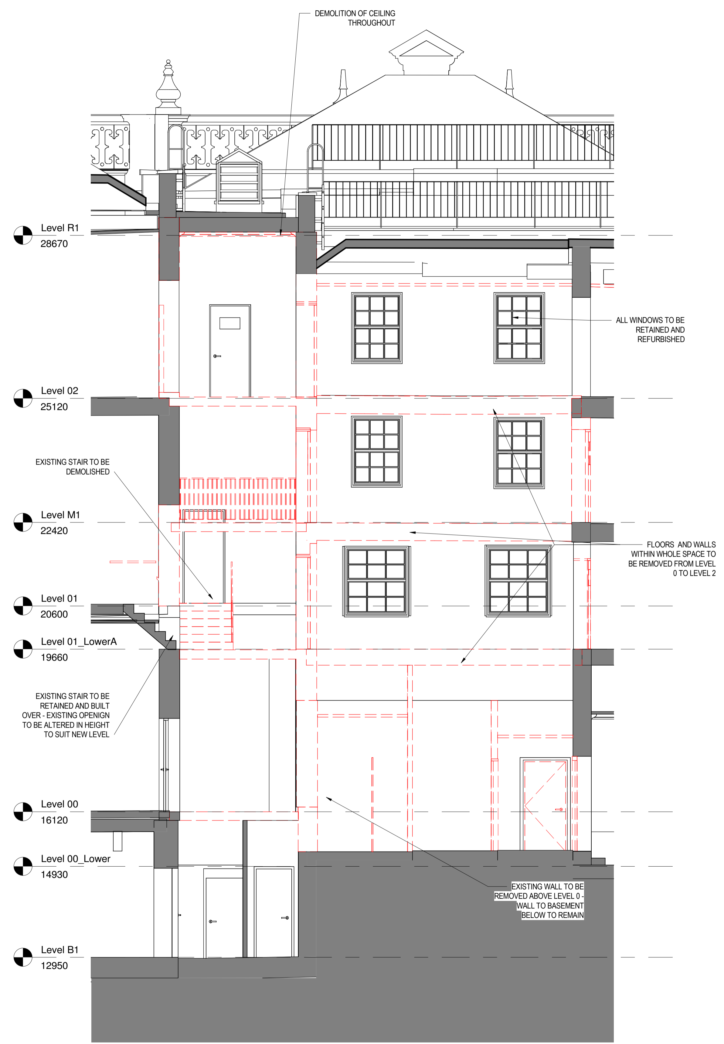
2 SECTION B STAIR - DEMOLITION 1 : 50
