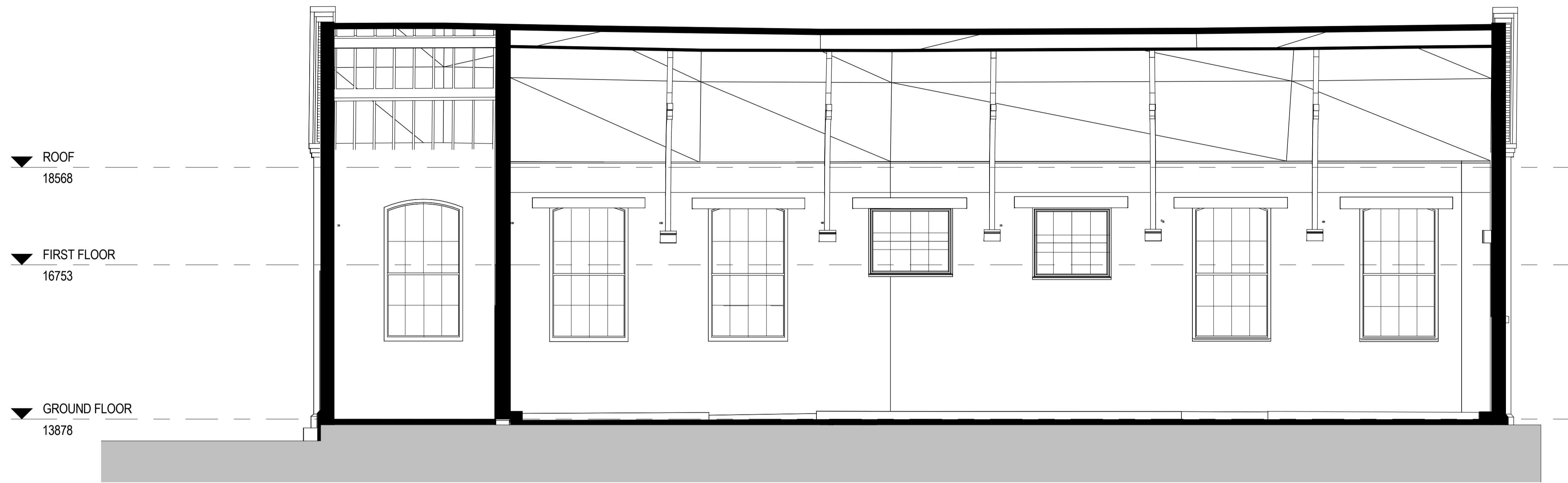
1 LONG SECTION AA - EXISTING 1 : 50
