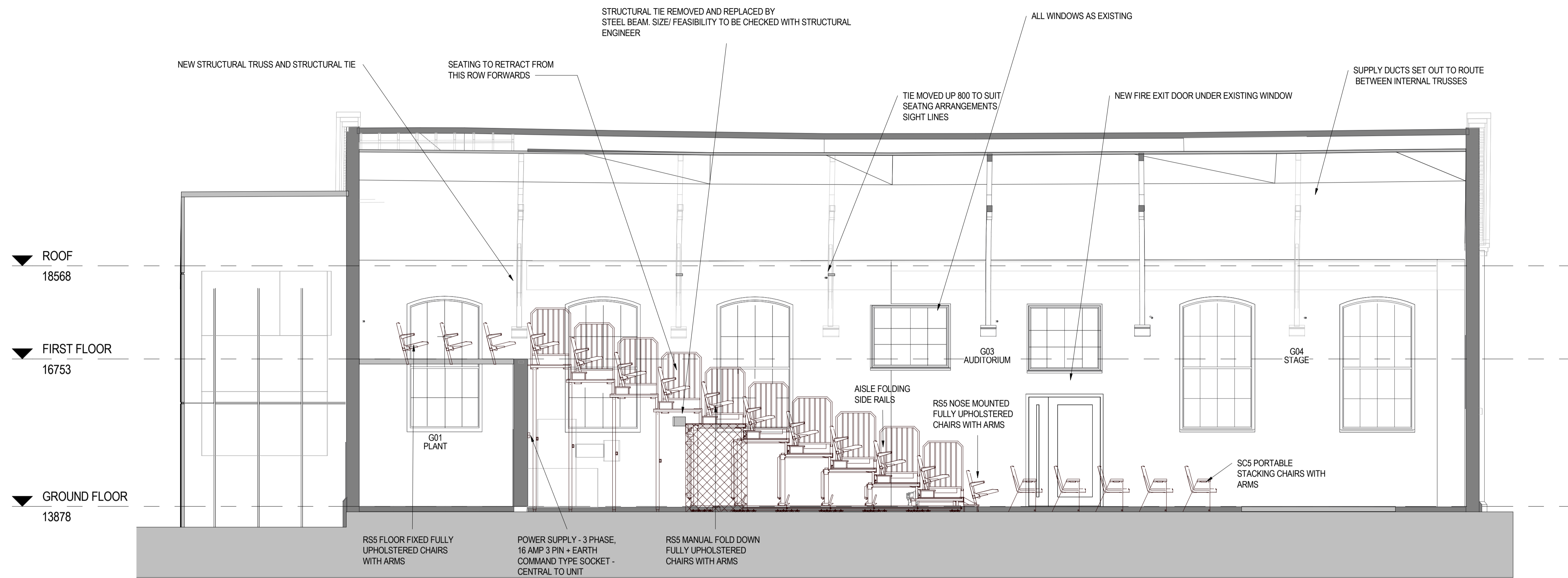
1 LONG SECTION AA 1 : 50
