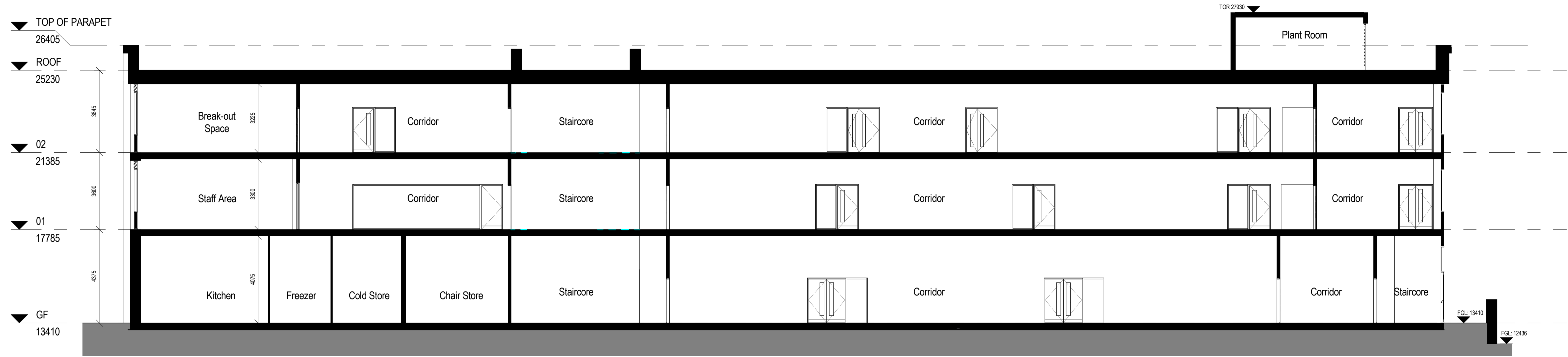
1 Section AA 1 : 100
