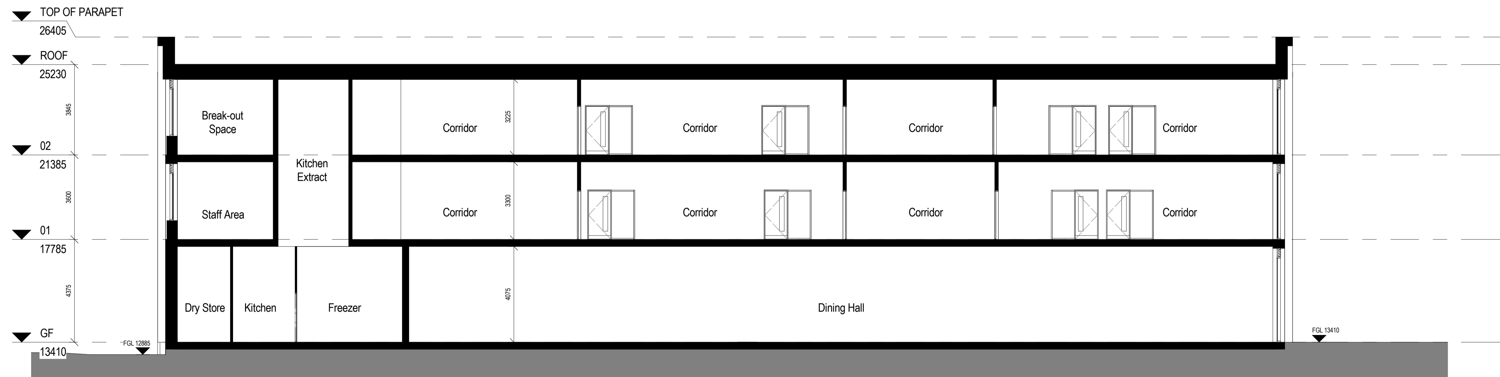
2 Section BB 1 : 100
