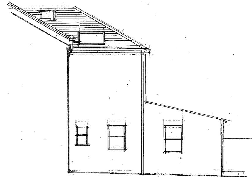
SIDE (SW) ELEVATION 1:100
