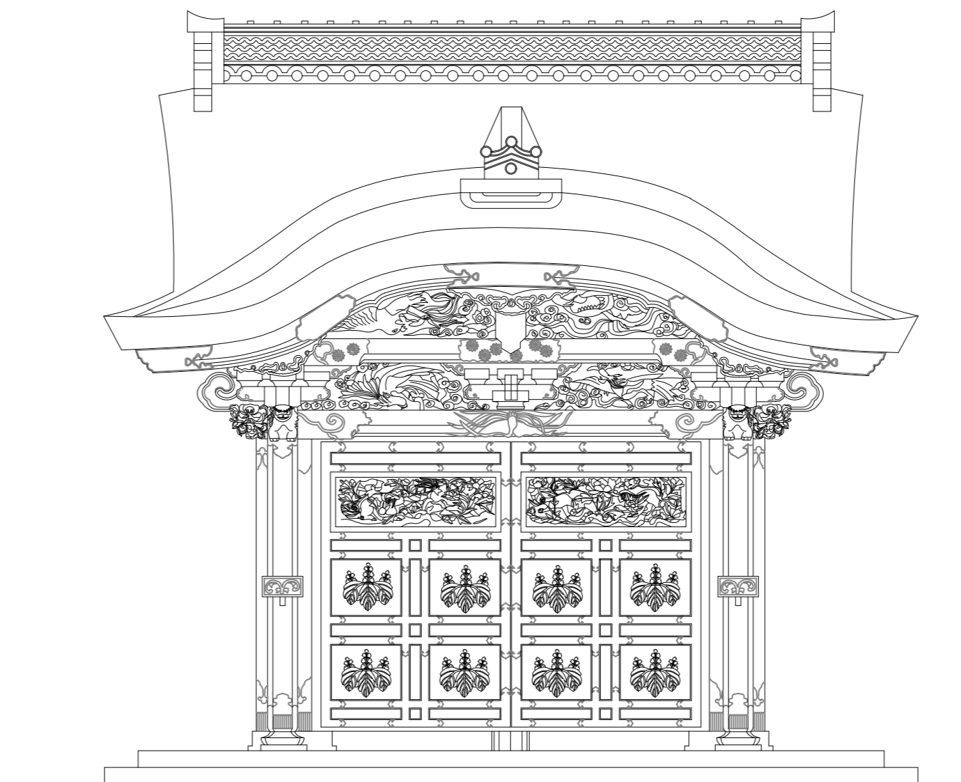
ELEVATION 3
