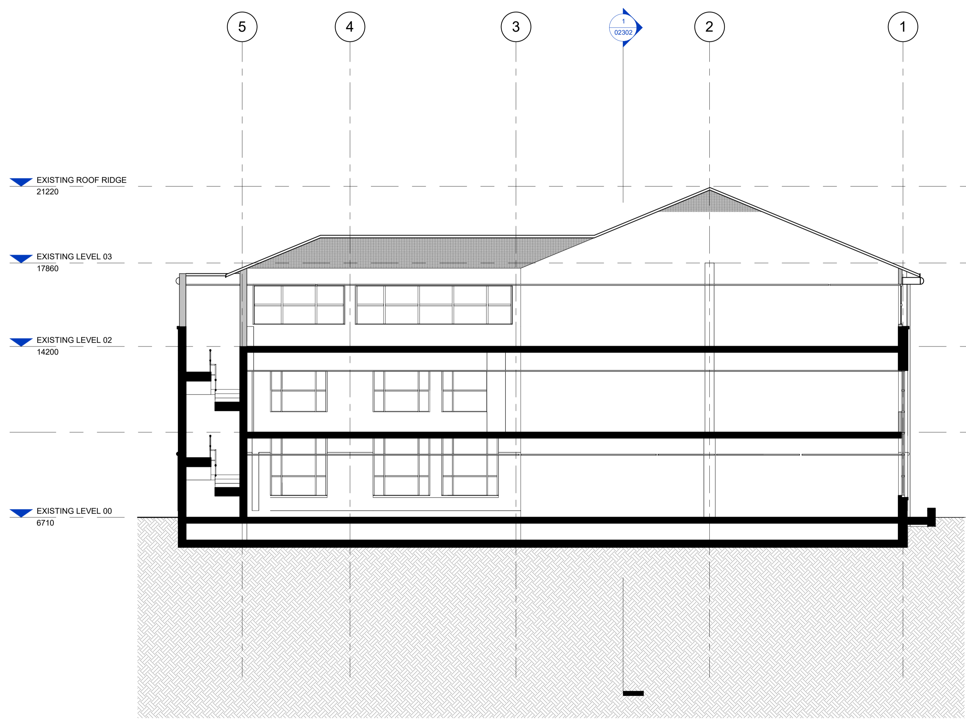
1 Existing Section A-A 1 : 100
