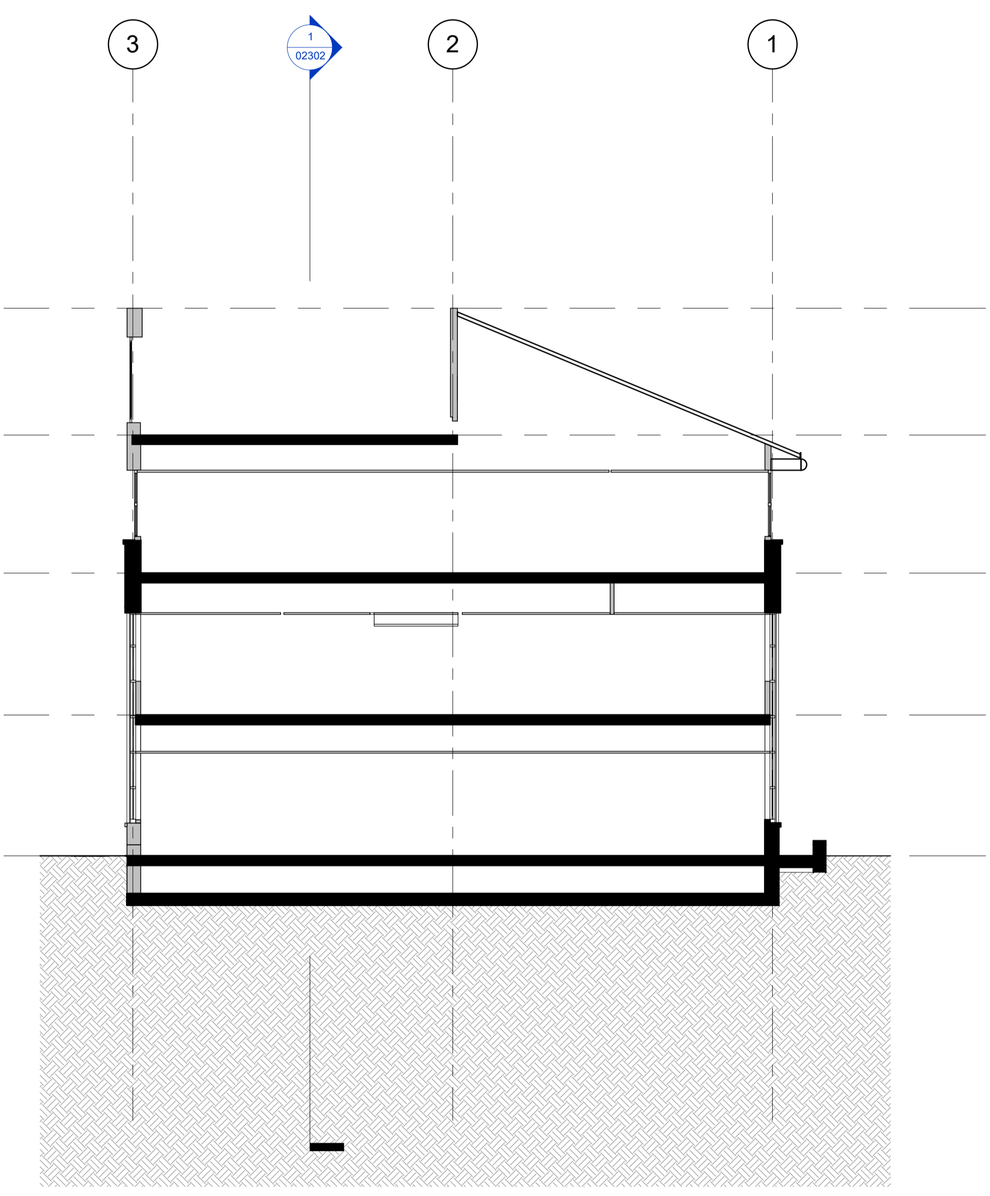
2 Existing Section B-B 1 : 100
