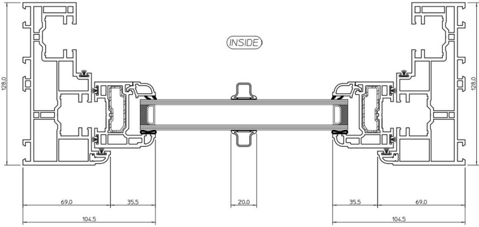
SECTION 'B-B'
