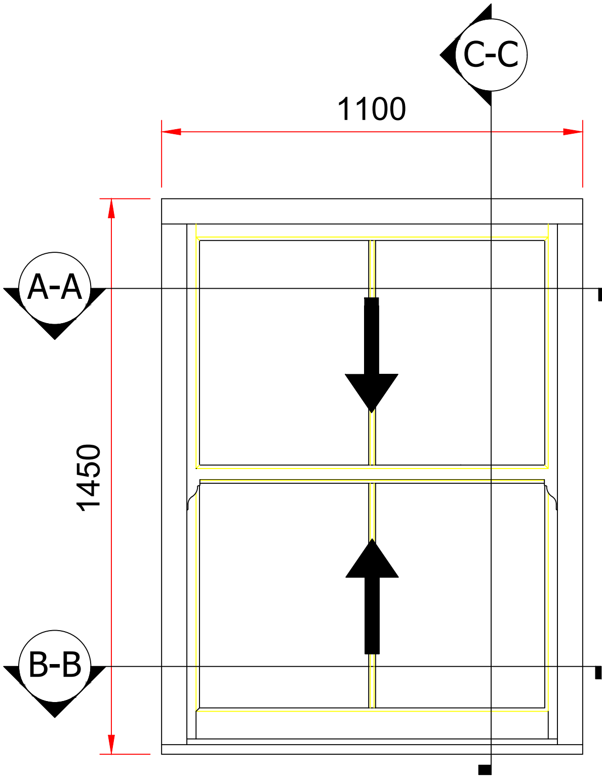
Frame No:1 Elevation
