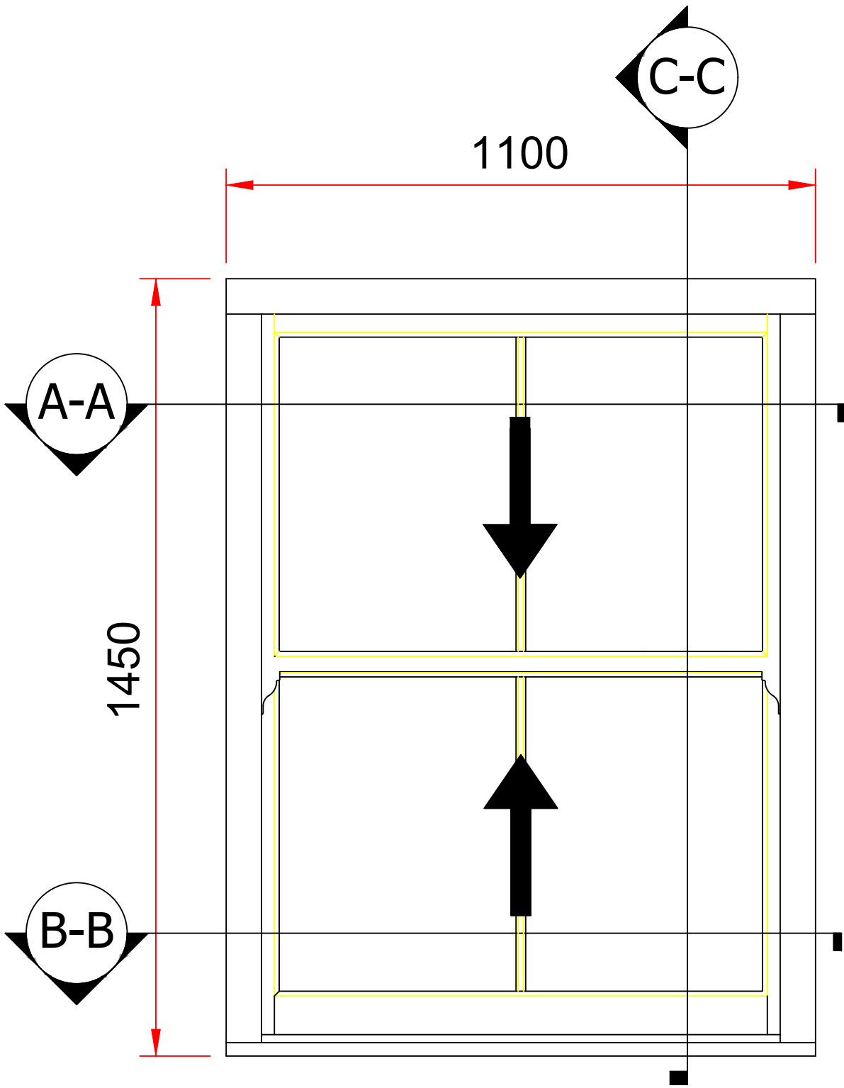
Frame No:6 Elevation
