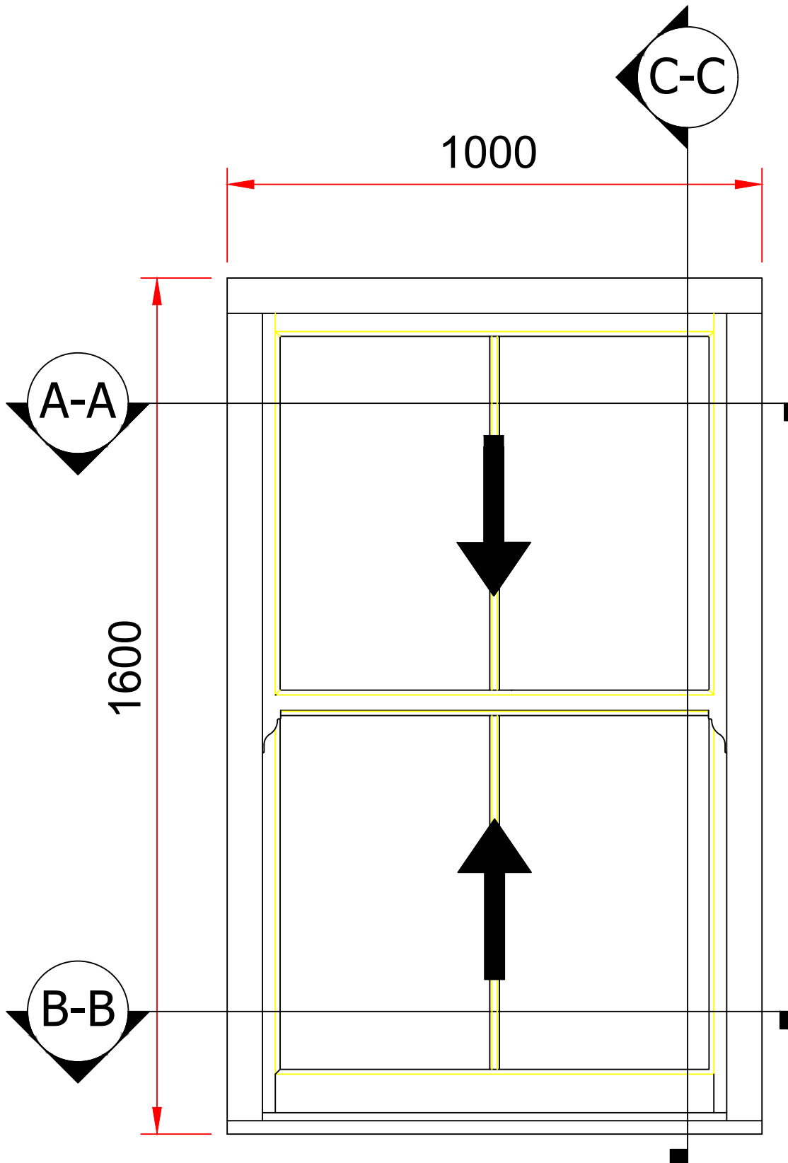
Frame No:3 Elevation
