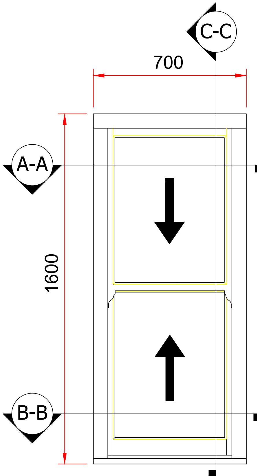
Frame No:2 Elevation
