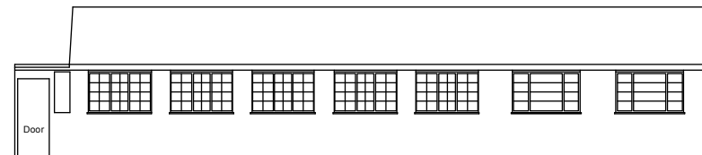
Elevation 2A
