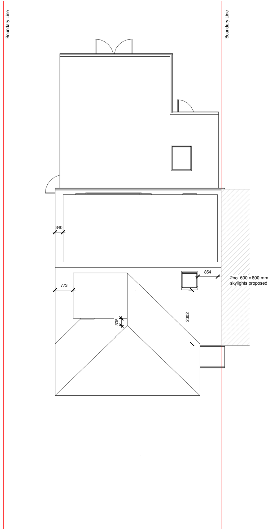
Roof Plan. 1 : 100
