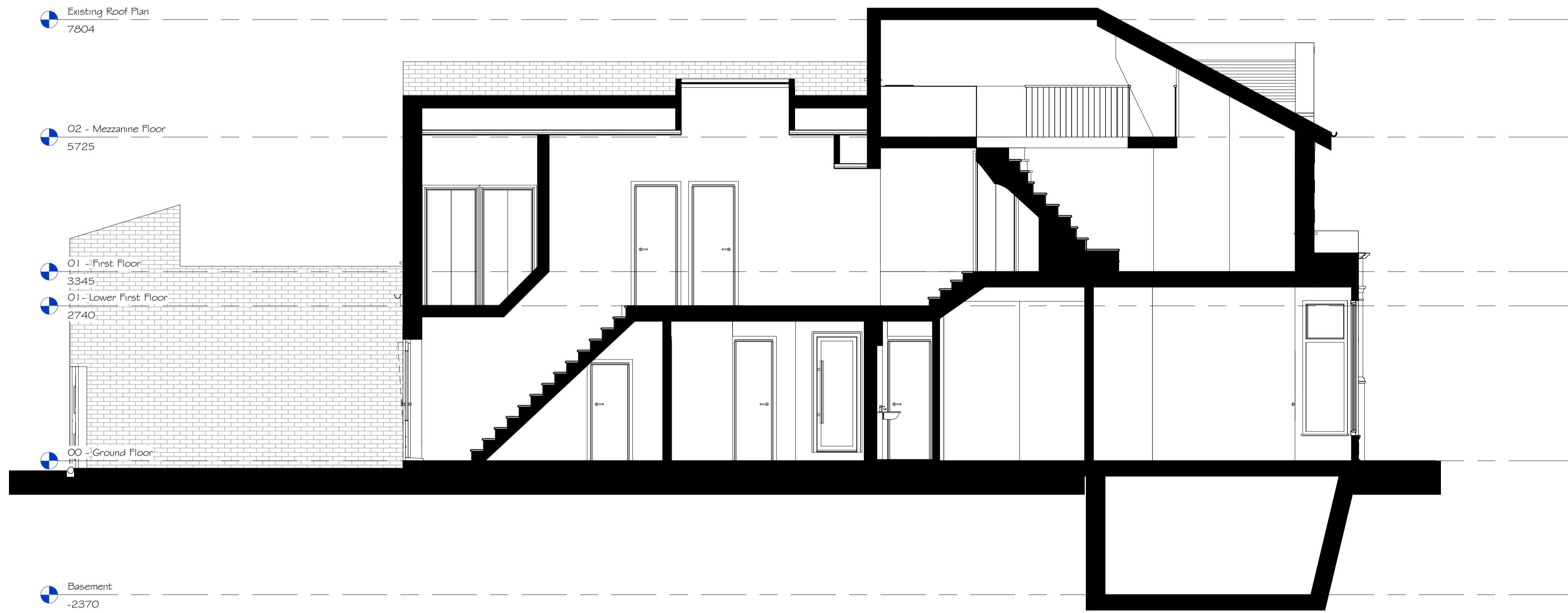
Existing Section 1 : 50
