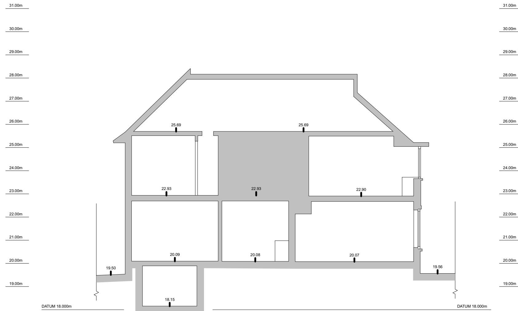
SECTION A-A
