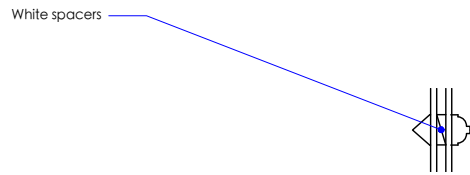
D2 - Glazing bar detail scale 1:5 @ A4
