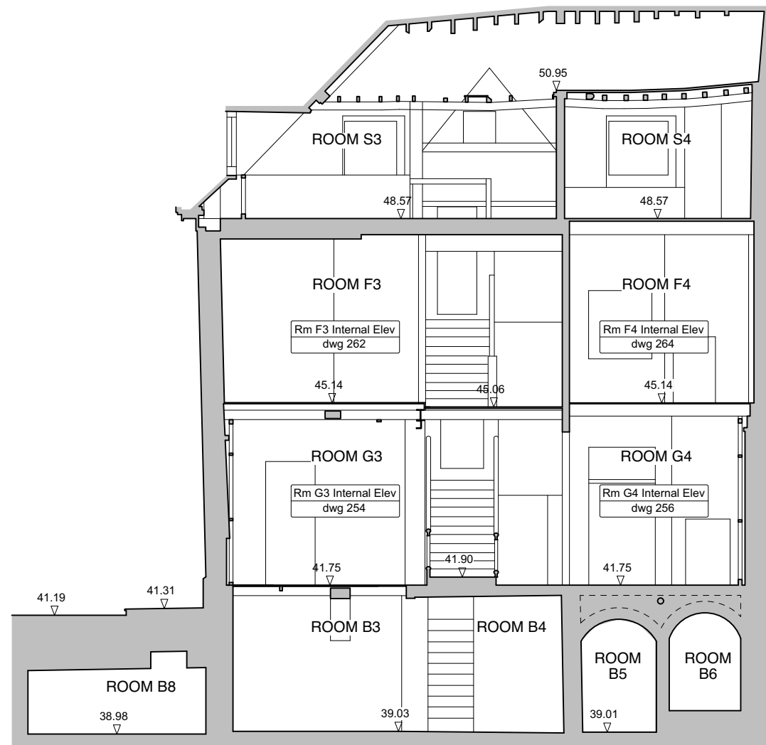
Section B-B : Existing
