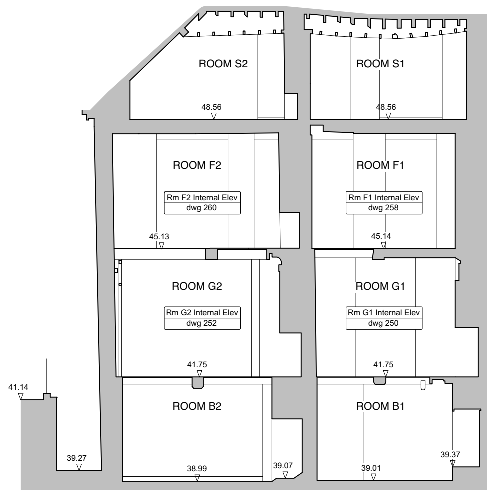
Section A-A : Existing
