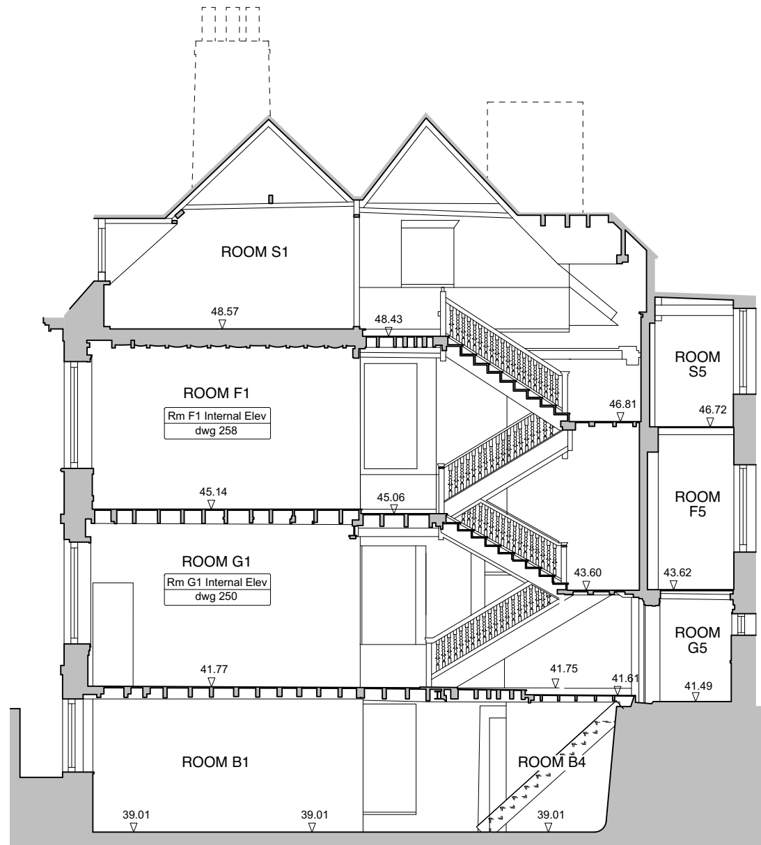
Section D-D : Existing
