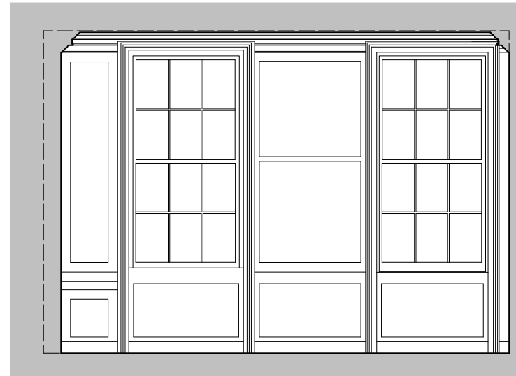
Elevation B
