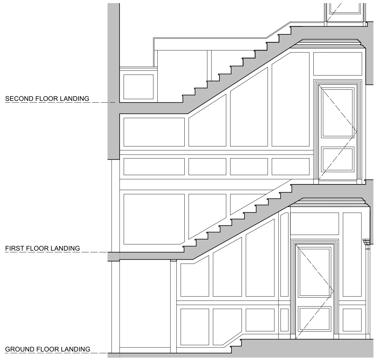
Elevation A
