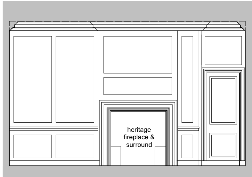
Elevation A
