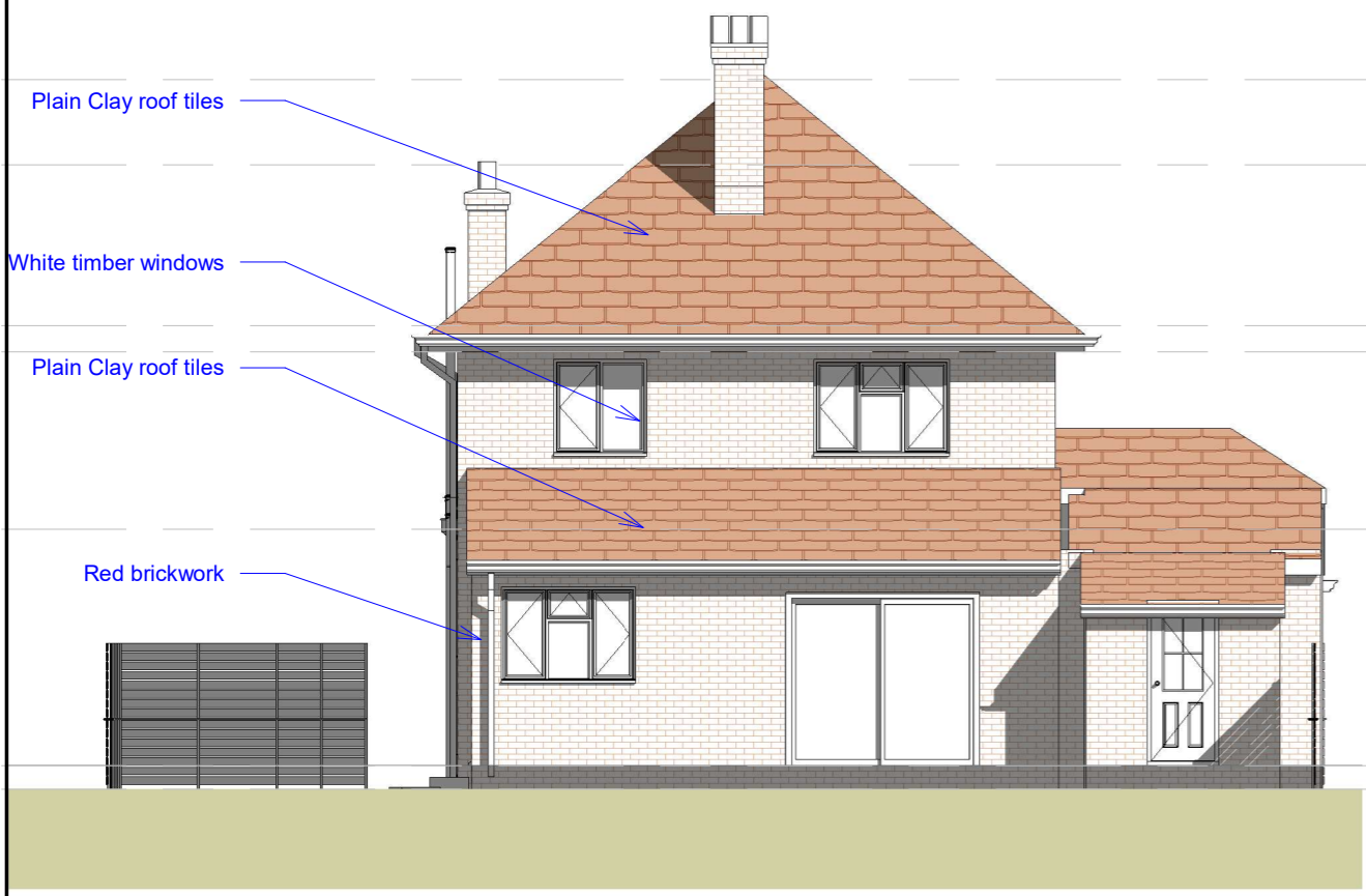
① Rear 1 : 100
