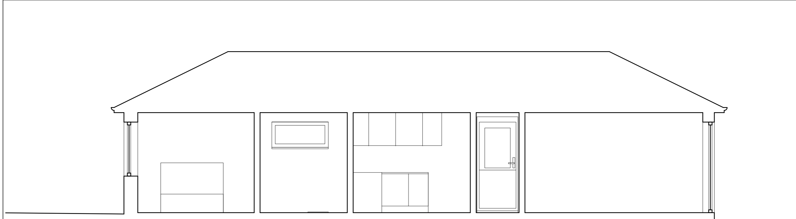
01 Long Section 1:50 at A3
