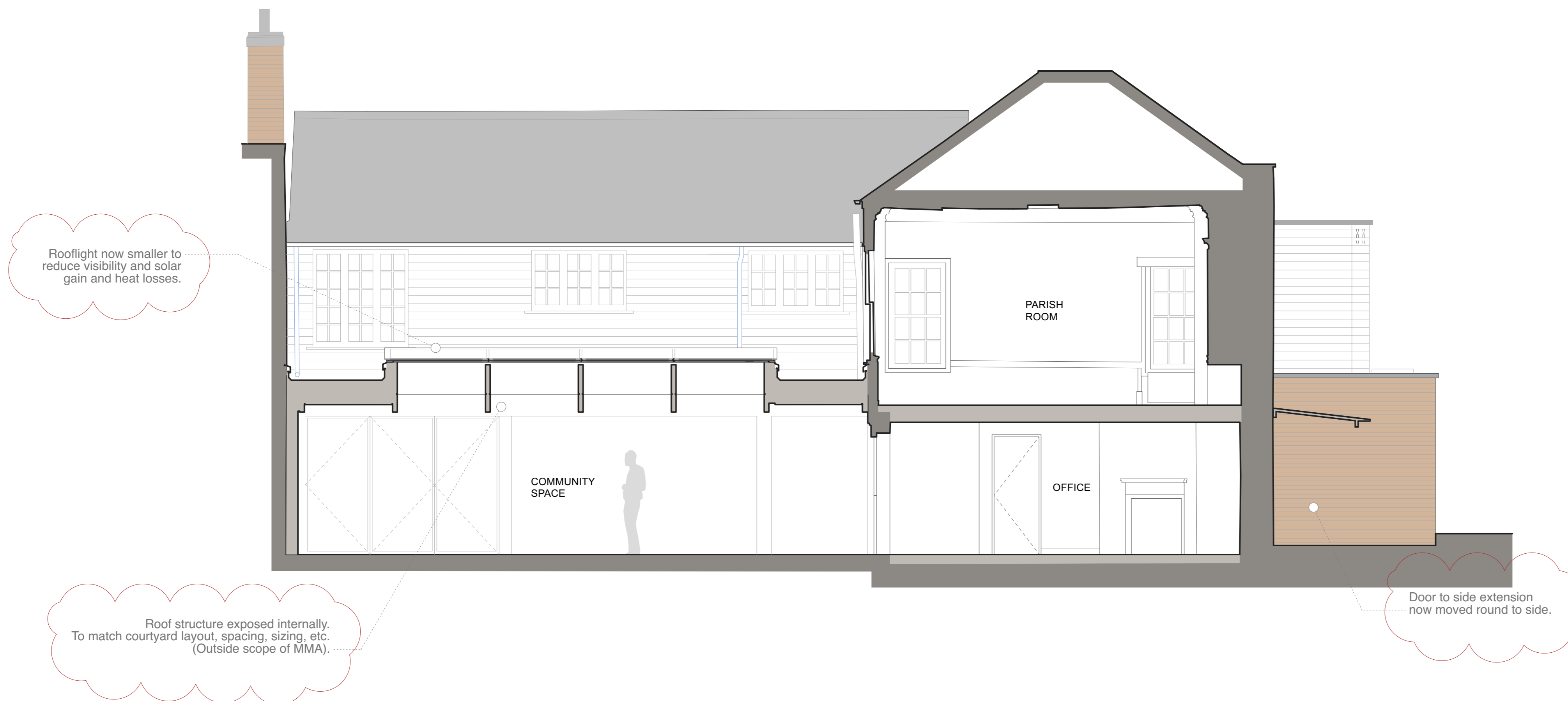
Section D-D
