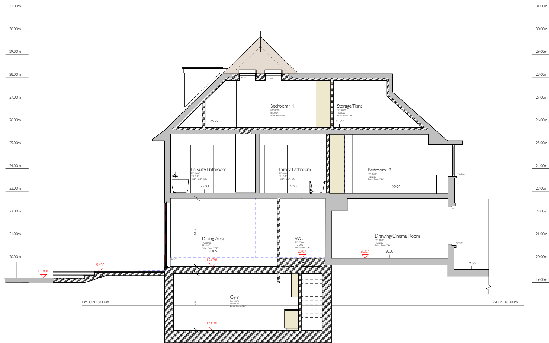
SECTION A-A
