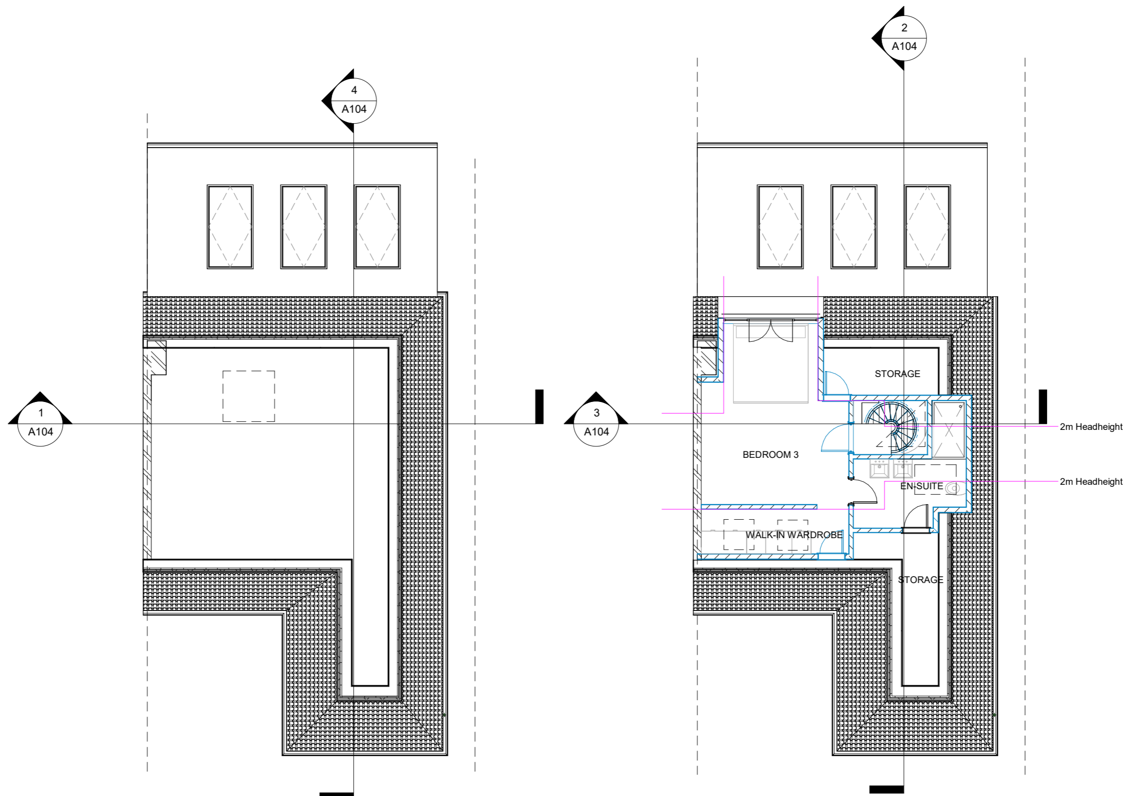
1 01- Existing 1 : 100
