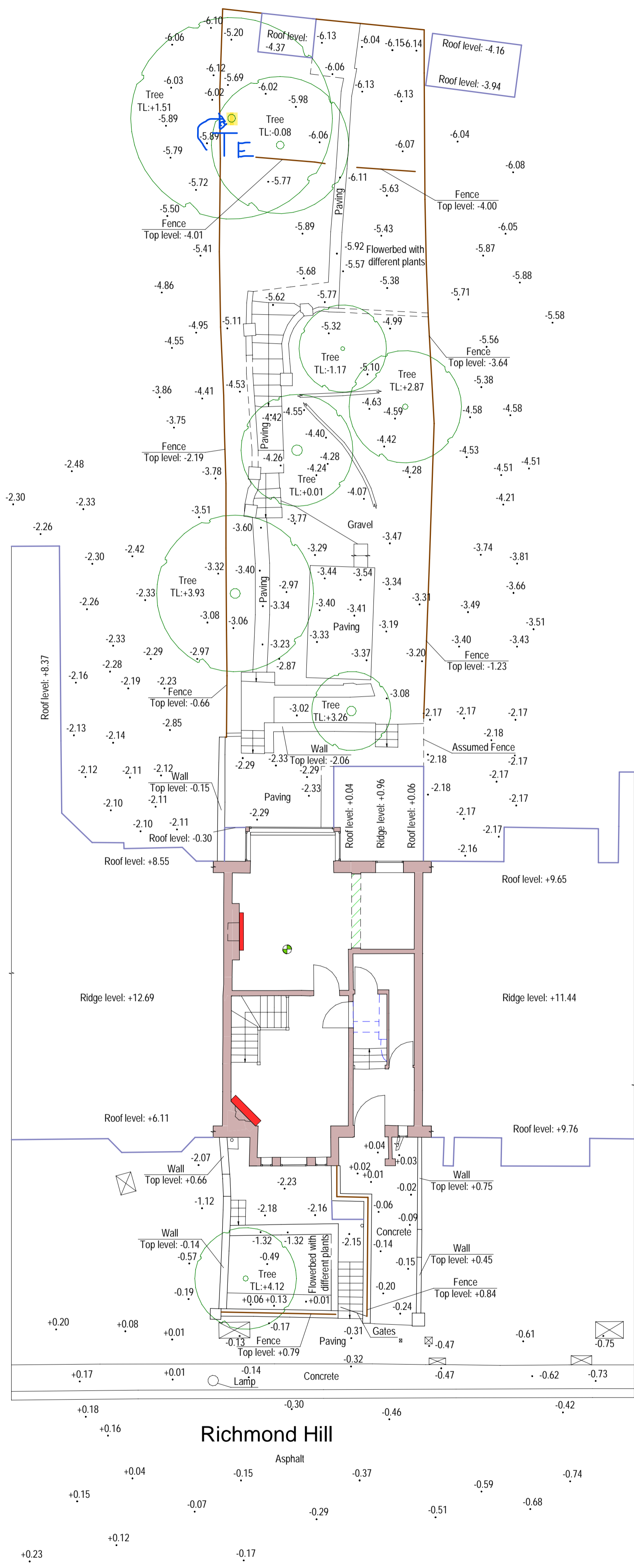
1 Existing site plan 1 : 100
