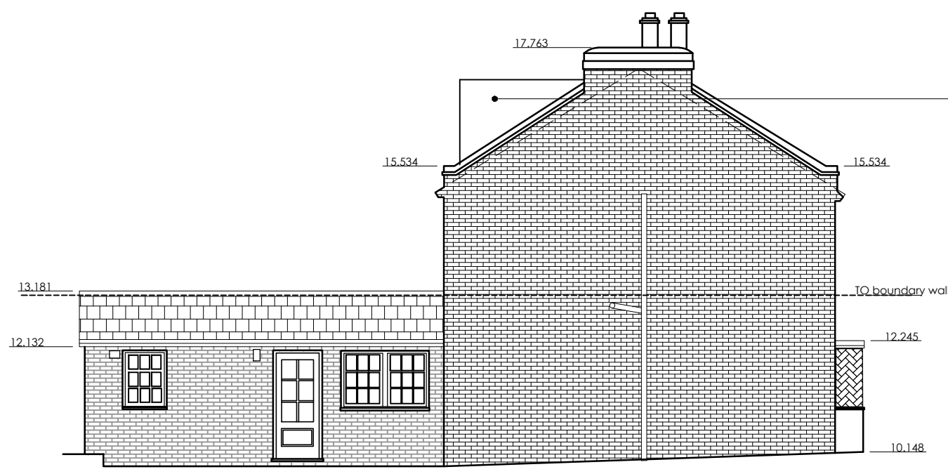
FLANK ELEVATION
