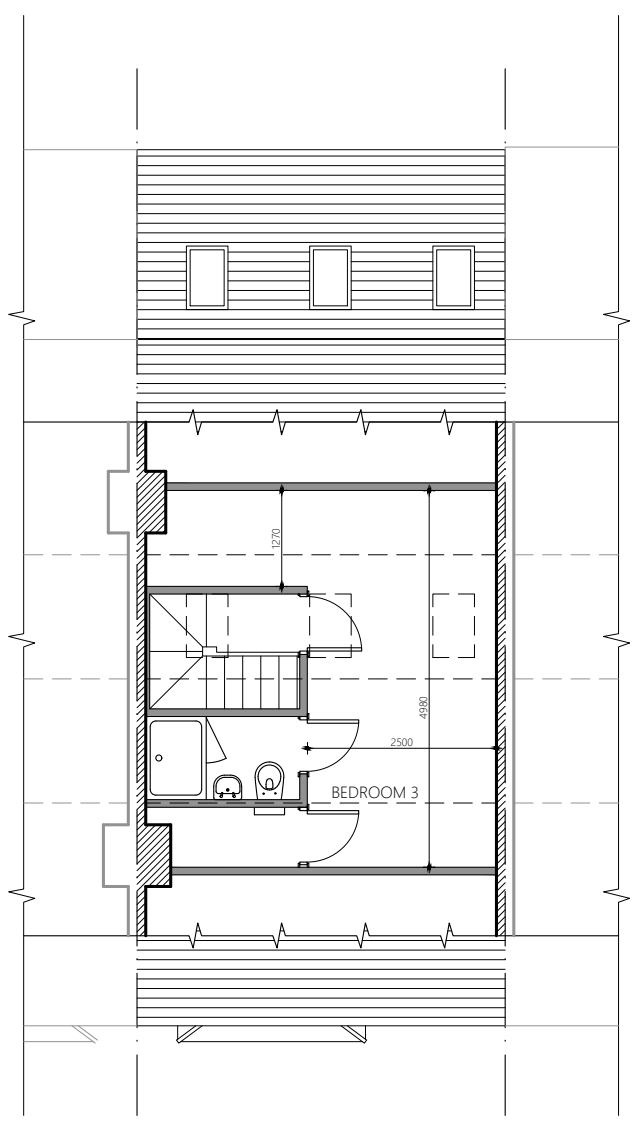
loft plan
