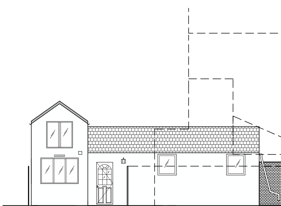
04 West Elevation D1001 SCALE: 1:100
