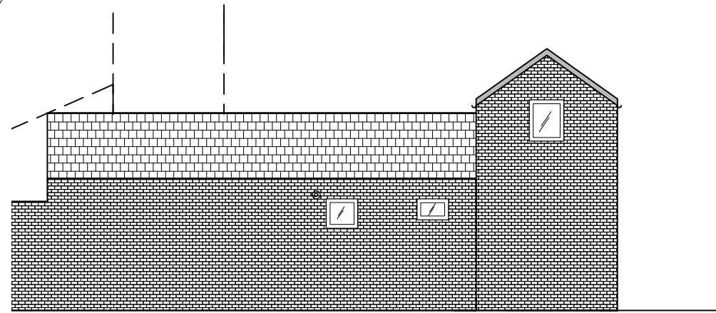
03 South Elevation D1001 SCALE: 1:100
