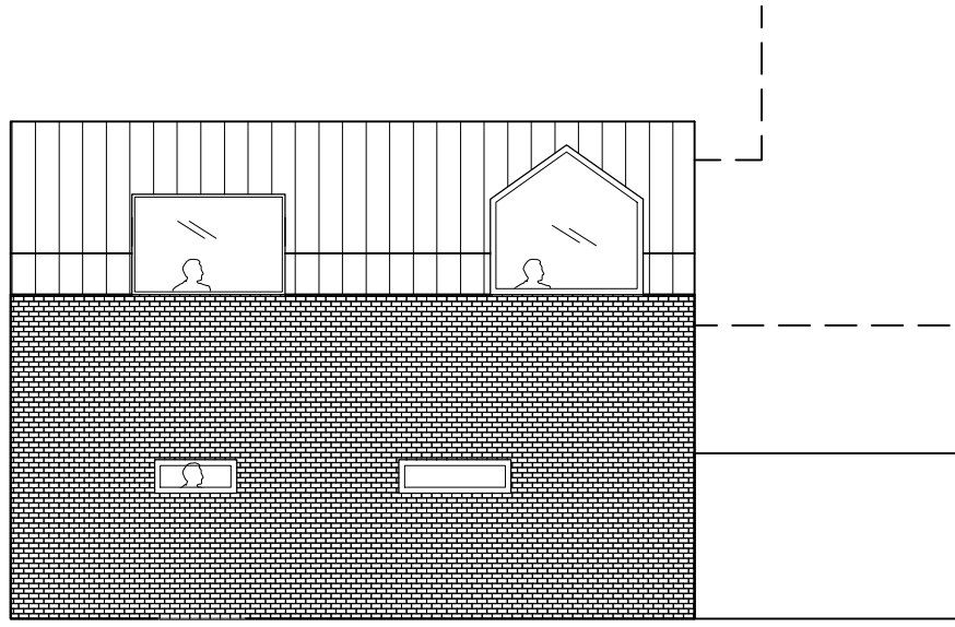
02 East Elevation D2001 SCALE: 1:100
