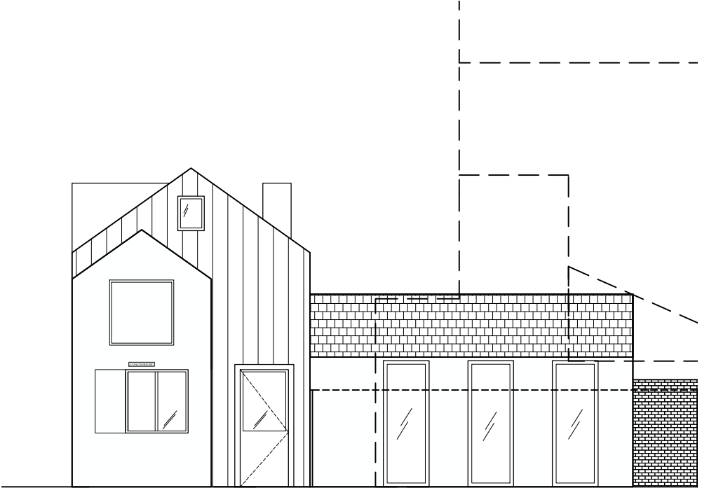
04 West Elevation D2001 SCALE: 1:100
