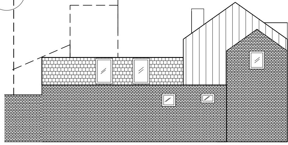
02 East Elevation D2001 SCALE: 1:100
